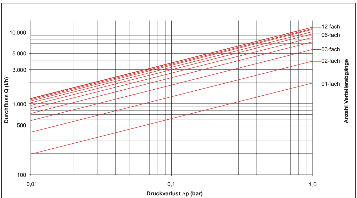
Diagramm 1 Durchfluss HKV 3000 Verteiler
